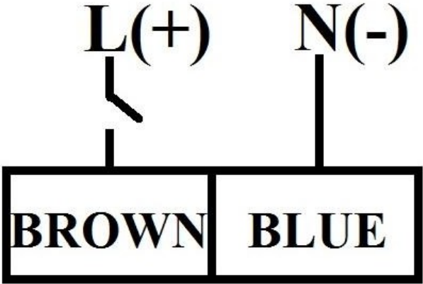
Схема управления шаровым краном с приводом AC220V; AC/DC24V с конденсатором:
